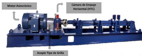
Figura 1. Sistema de bombeo horizontal (Hpump).
