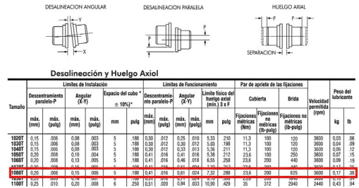
Figura 3. Límites de funcionamiento del acoplamiento utilizado.
