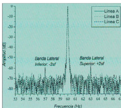
Figura 5. Ejemplo de un espectro de frecuencia para análisis del rotor.
